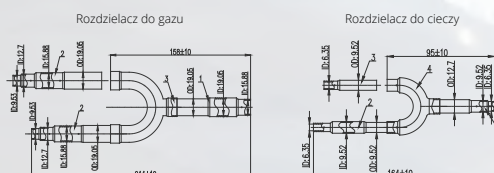
Rozdzielacze RVF-RDIX17
